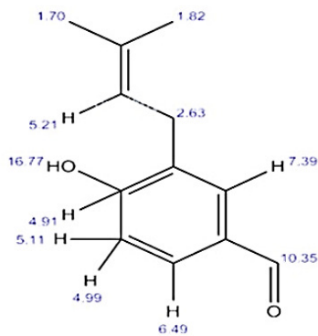
Figure-6. 4-hydroxy-3-(3-methylbut-2-enyl) benzaldehyde
